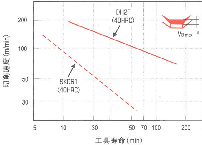
● 端铣工具寿命图
