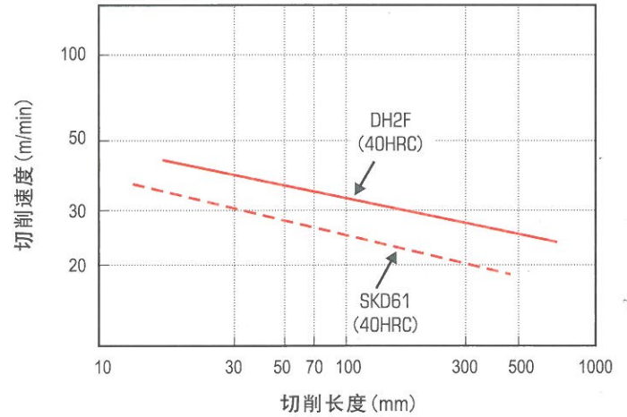
● 高速钢钻头工具寿命图
